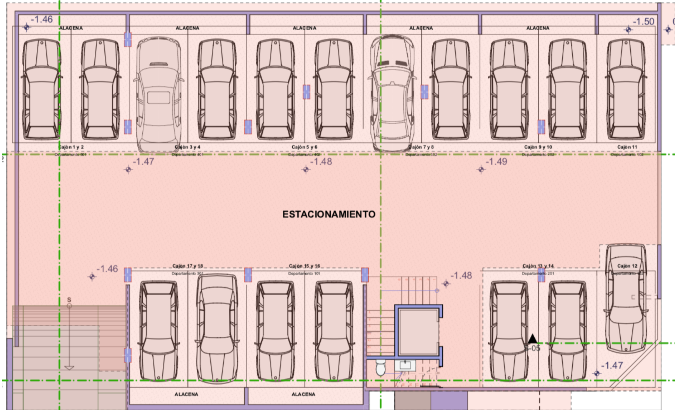
PLANTA SOTANO
